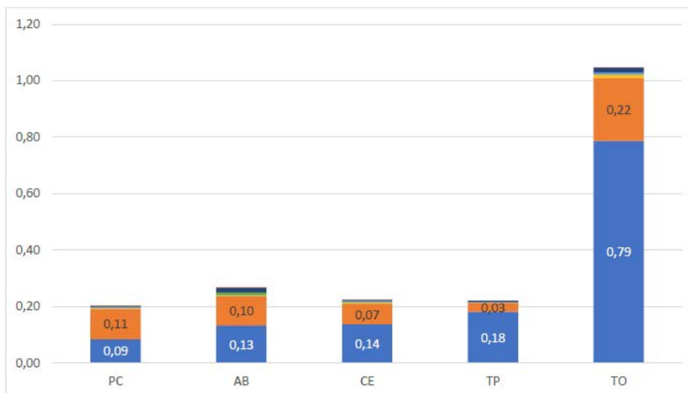
Figura 5: Gráfico do FD médio por região da fachada - paredes contínuas (PC), aberturas (AB), cantos e extremidades (CE), transição entre pavimentos (TP) e topo (TO).
